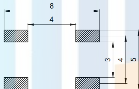
PCB. 焊接图
