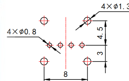
印制线路板图
