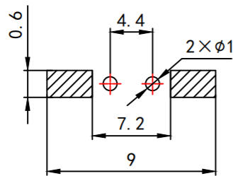
PCB. 焊接图
