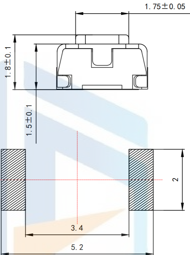
PCB. 焊接图
