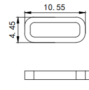
防水圈图示
