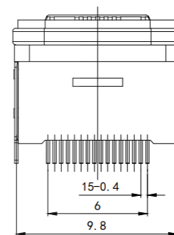
装前塞示意图
