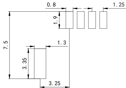
安装开孔尺寸
